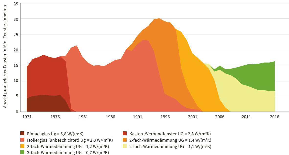
Abb. 4: Produzierte Fenster nach Verglasungsart
