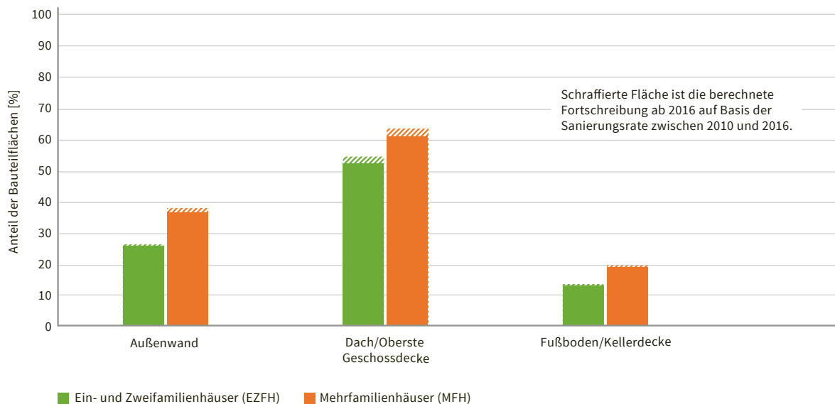
Abb. 3: Nachträgliche Wärmedämmung im Bestand nach Bauteilen und Gebäudeart
