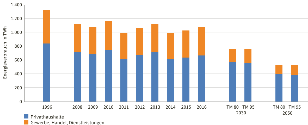
Abb. 19: Gebäudeenergiebedarf 2030/2050
