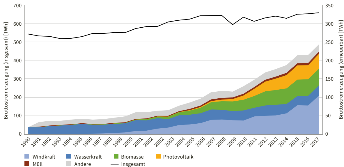
Abb. 13: Erneuerbare Energien in der Stromerzeugung
