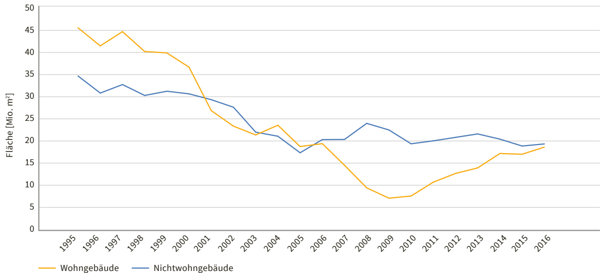
Abb. 9: Entwicklung neue Wohn- und Nutzfläche
