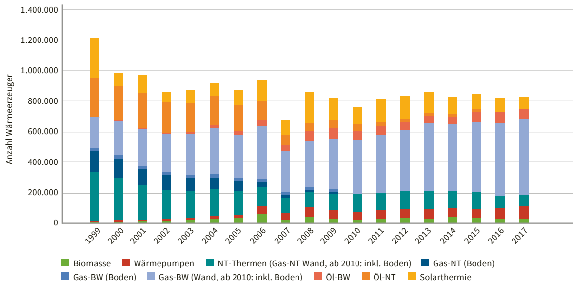
Abb. 2: Absatzzahlen von Wärmeerzeugern
