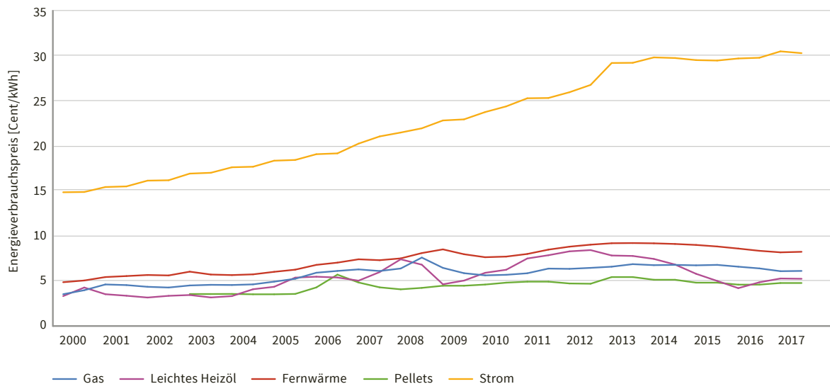
Abb. 18: Verbraucherpreise für Heizenergie nach Energieträger
