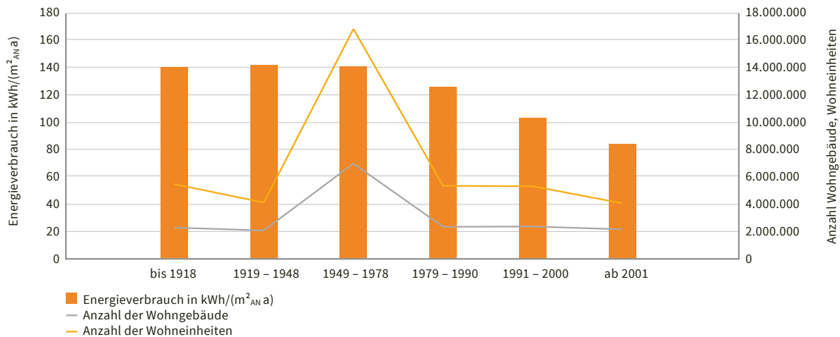
Abb. 1: Energieverbrauch des Wohngebäudebestandes
