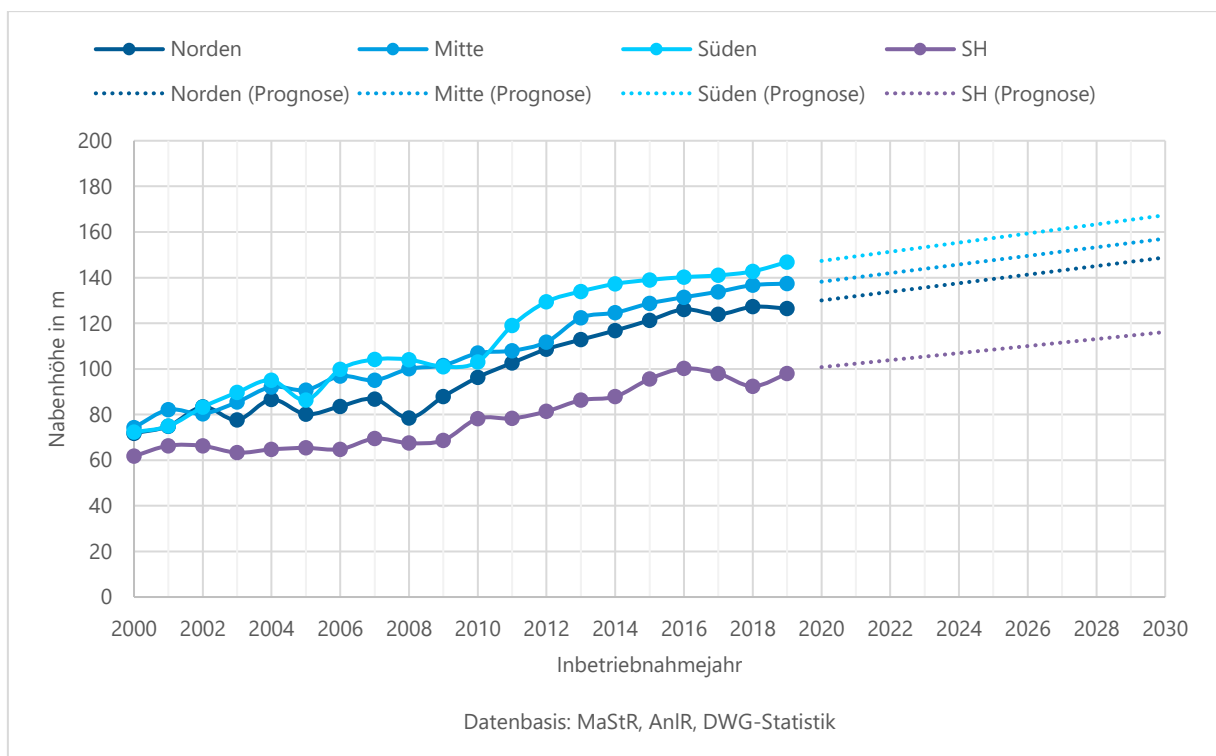
Abbildung B: Prognose für die Entwicklung der mittleren Nabenhöhe
