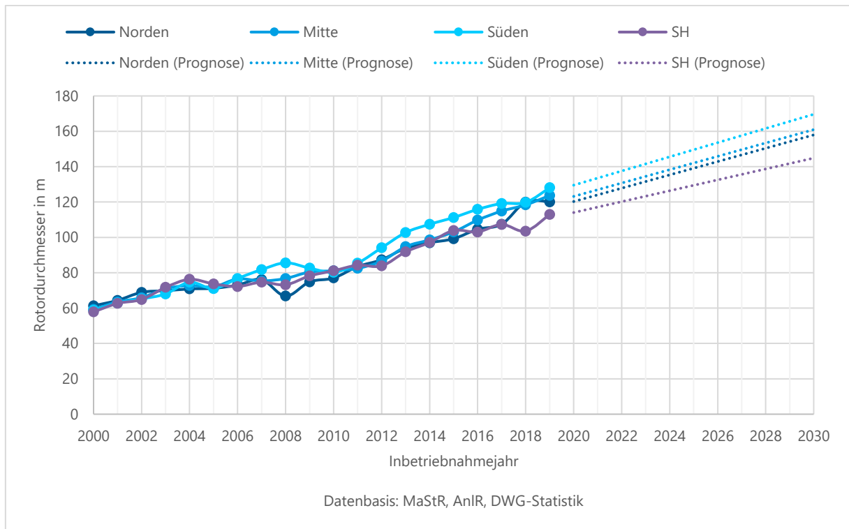
Abbildung A: Prognose für die Entwicklung des mittleren Rotordurchmessers
